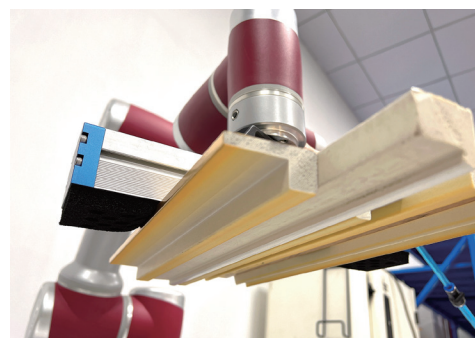
* 海绵吸具HVGP吸取异形木条
